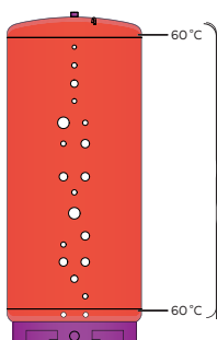
Bereitchaftszone: 60°C
