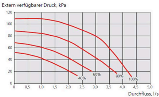
Quellenkreispumpe (im Lieferumfang)
